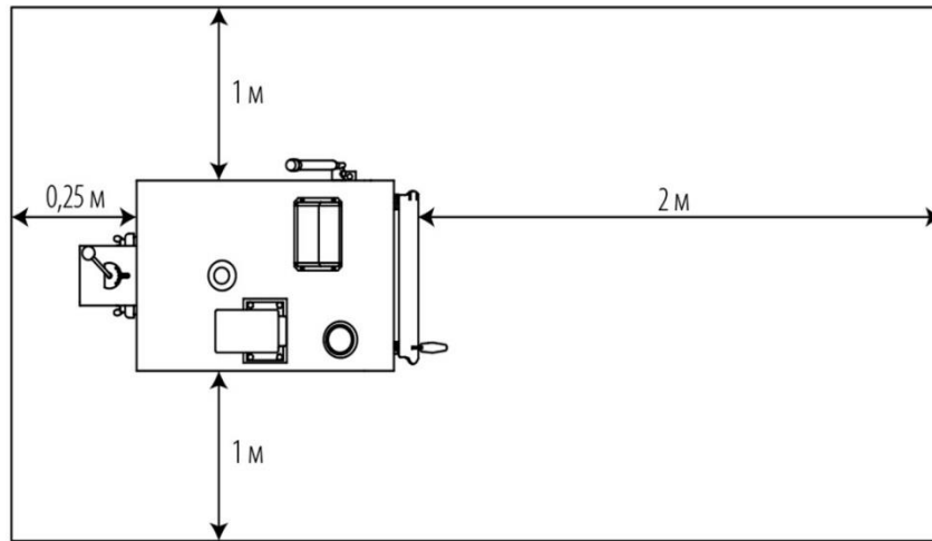
Рис. 1. Наглядное расположение котла в котельной.
