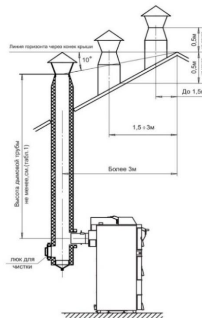
Рис 2. Вариант установки дымохода.
